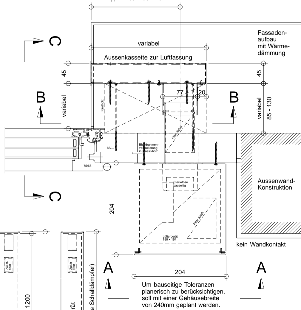
Grundriss
