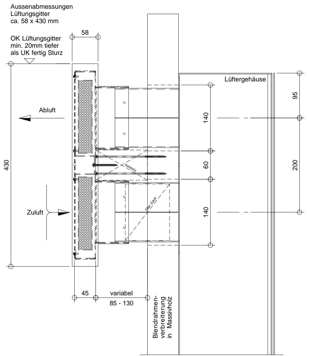
Schnitt C - C
